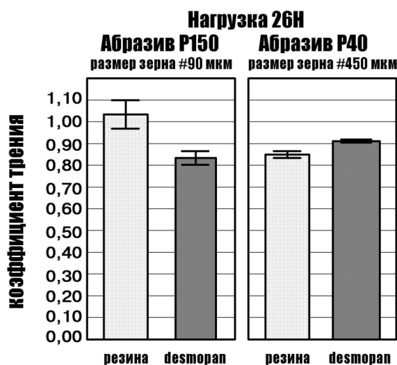
Рисунок 3 – Коэффициент трения материалов во время теста
